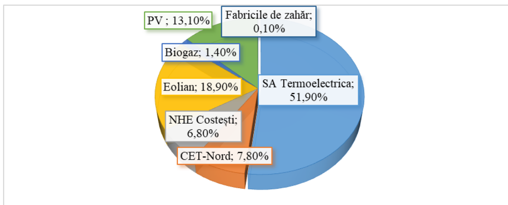
Figura 2. Structura producerii locale de energie electrică din Republica Moldova, în anul 2023
